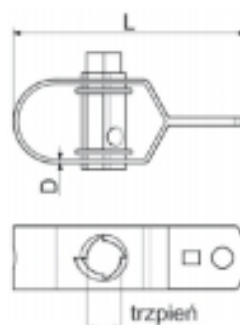
NACIĄG DO DRUTU (OCYNK GALWANICZNY)
